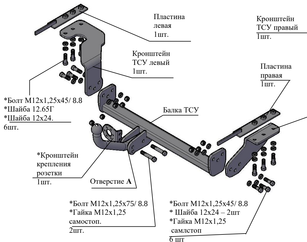
Рис.1 Тягово-сцепное устройство 7711
