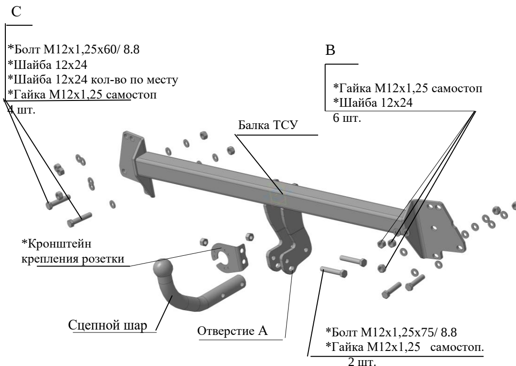
Рис.1 Тягово-сцепное устройство ТСУ 7880.
