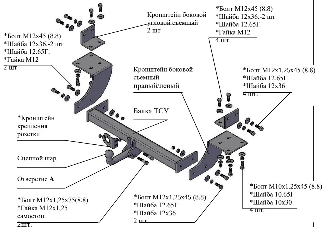
Рис.1 Тягово-сцепное устройство 9460
