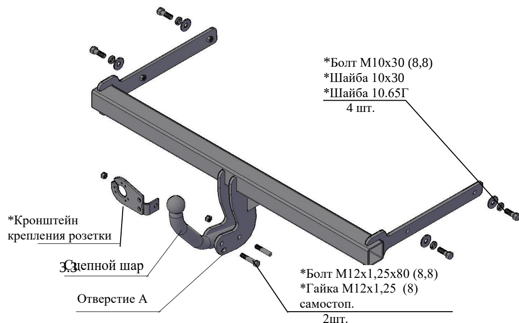
Рис.1 Тягово-сцепное устройство ТСУ 9710.
